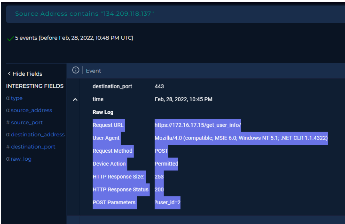
Figura 4: Evidencia del acceso no autorizado con estado HTTP 200.
